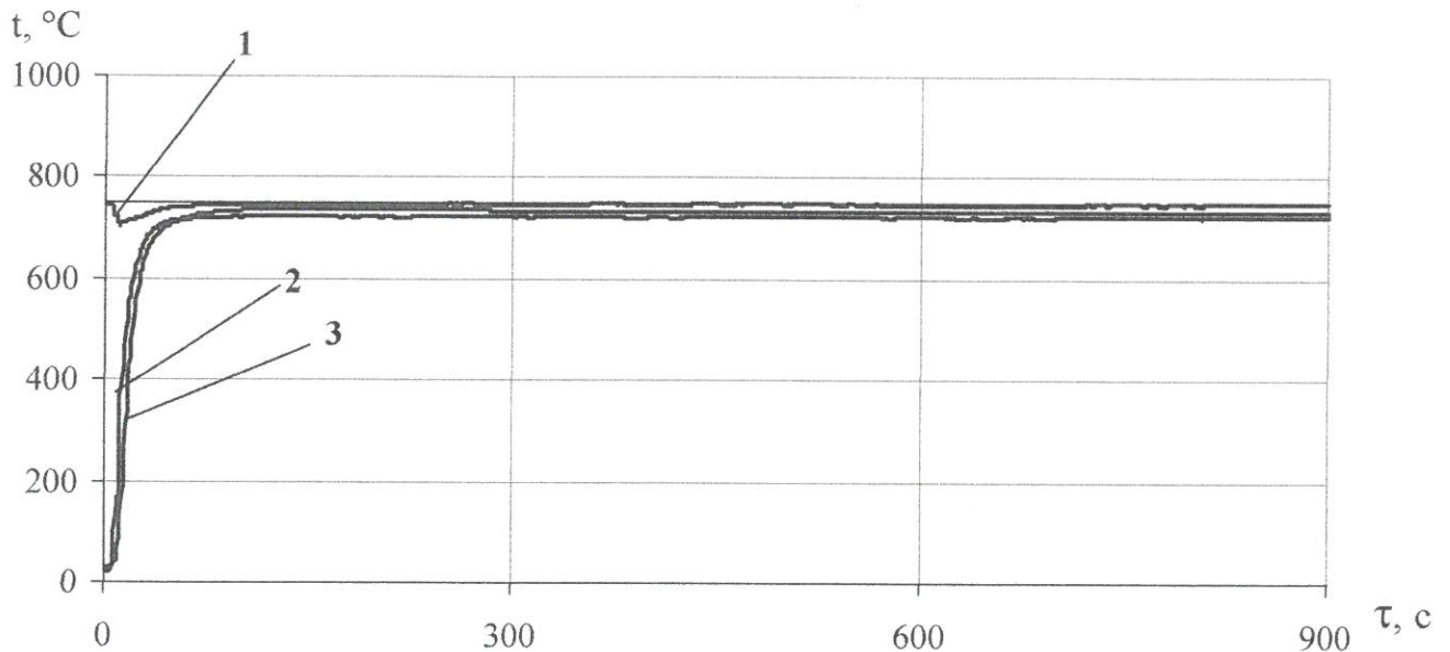
Рисунок 1 - Характерний графік змінення температури у печі (1), на поверхні (2) та всередині (3), зразків під час випробувань виробів тепло-звукоізоляційних зі скляного штапельного волокна, марки ЕКО-ДАХ, виробництва ТОВ «УРСА Євразія» (Росія).
